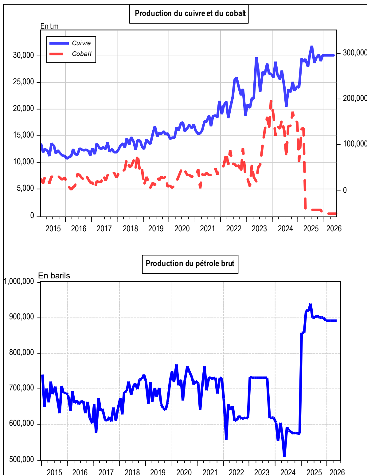
Graphique II.1 : Evolution des principales productions minières et pétrolière
